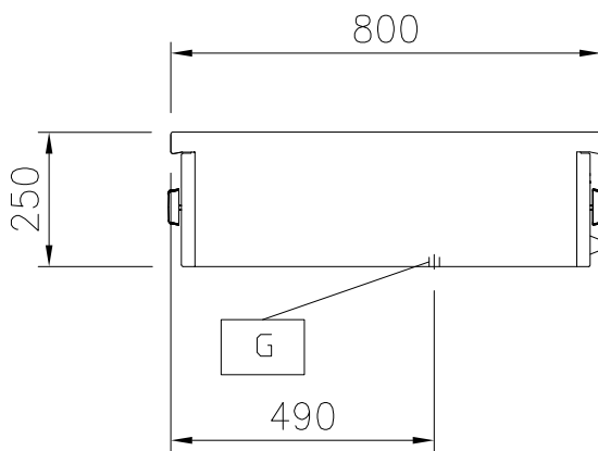
Zij aanzicht
